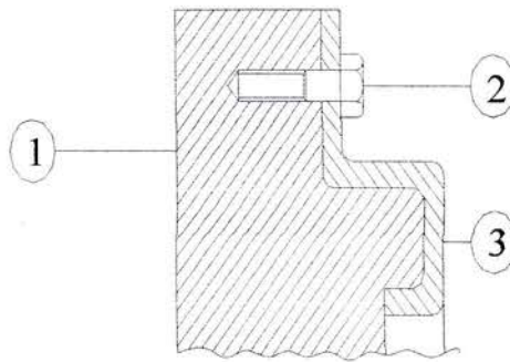
Gambar 9. 3. Baut Pengikat Penutup Kopling
