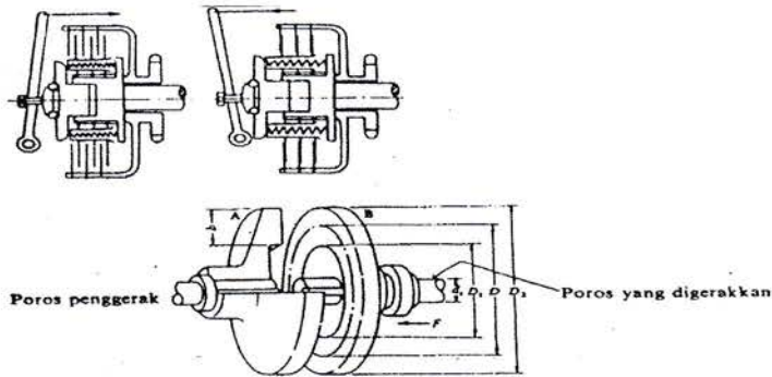
Gambar 2.12. Kopling Piat
