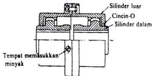
Gambar 2.7. Kopling Gigi
