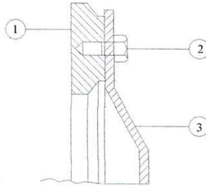
Gambar 9. 2. Baut Pengikat Pegas Matahari Dengan Plat Penekan
