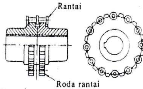
Gambar 2.8. Kopling Rantai
