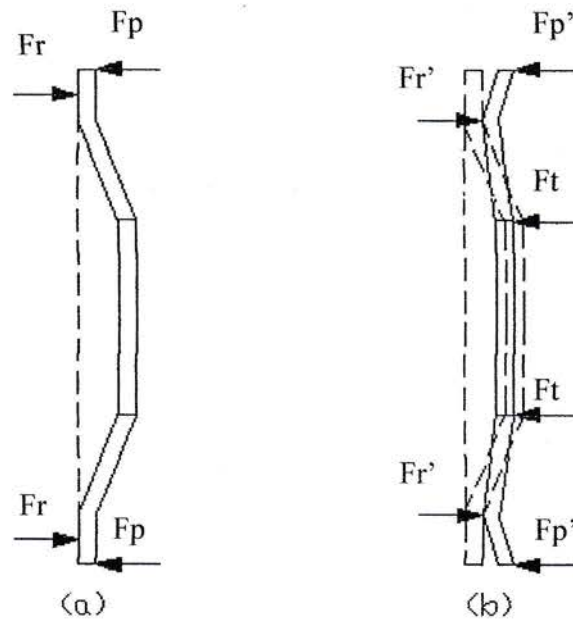
Gambar 8. 2. Diagram gaya-gaya yang bekerja pada pegas
