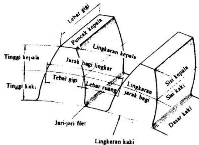
Gambar.3.1.Roda Gigi
