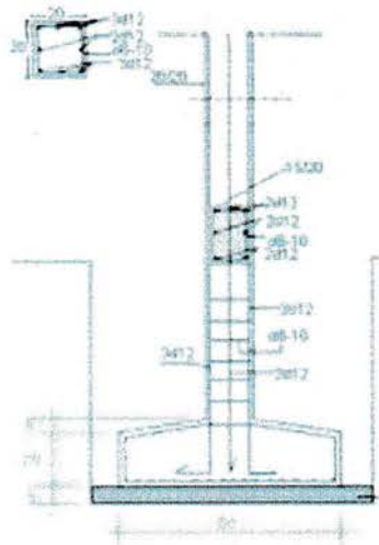
Gambar : Pondasi plat dan kolom untuk bangunan lantai 2
